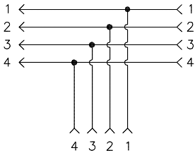
WIRING SCHEMATIC
